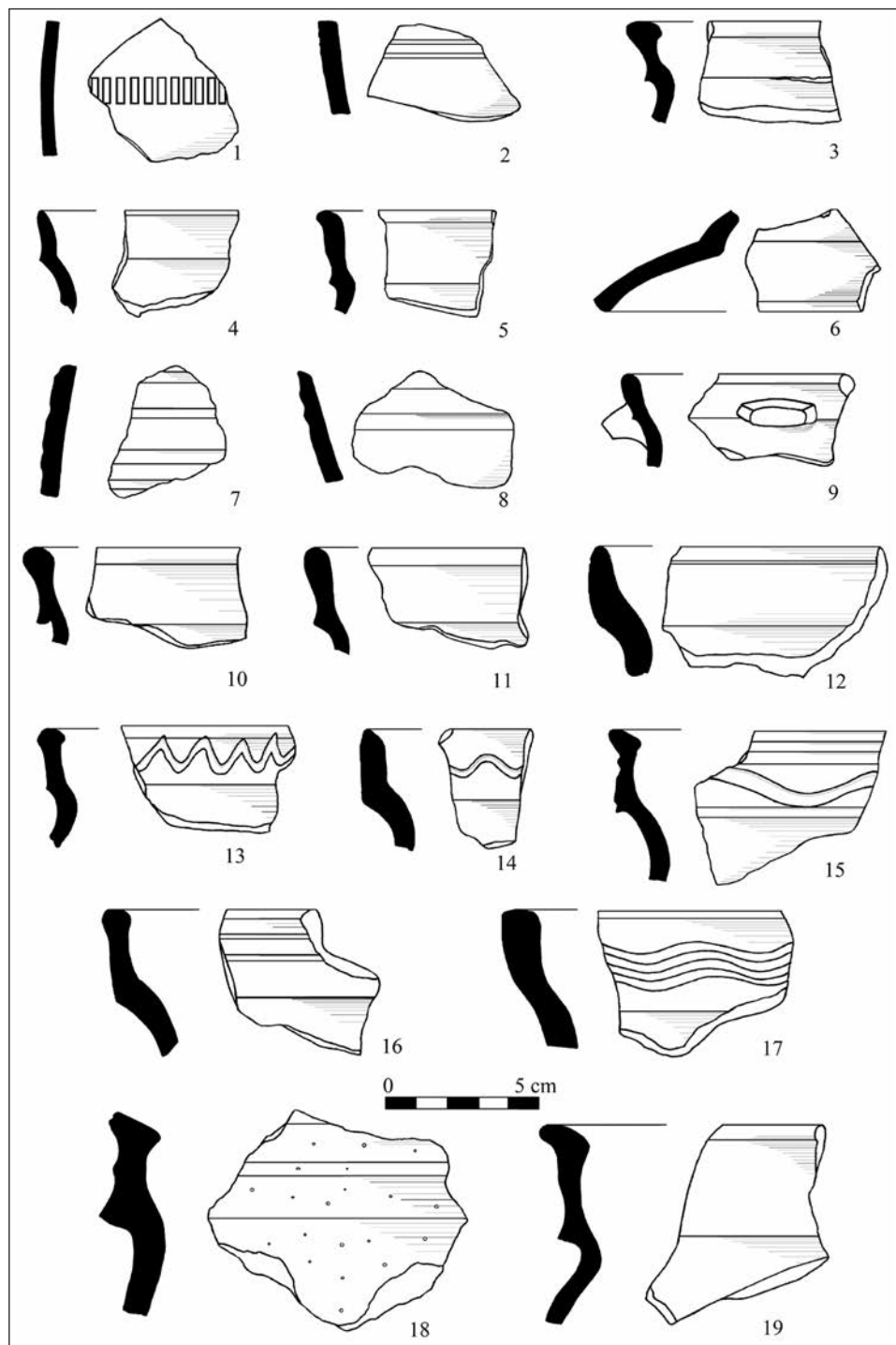
Výběr keramických nálezů z vrcholného středověku ze zahrady domu Staromajetinská č. p. 14. Kresba Lukáš Hlubek. V textu je na tuto keramiku odkazováno číslem obrázku 8.
